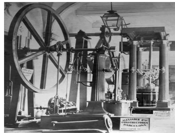
5. L'espai d'Alexander Hermanos en l'Exposició Catalana de 1877.
