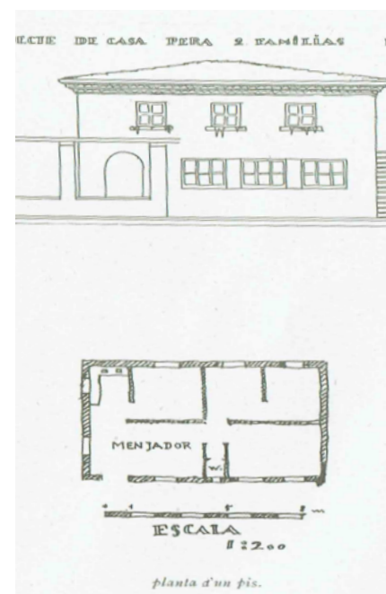
39. Projecte de Les cases a bon preu (1920). Casa de dues plantes.
