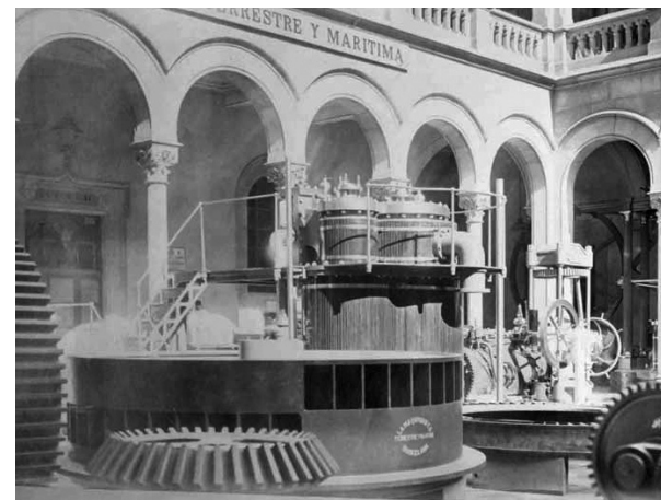
4. Una de les màquines exposades al claustre de la Universitat de Barcelona en l'Exposició Catalana de 1877.
