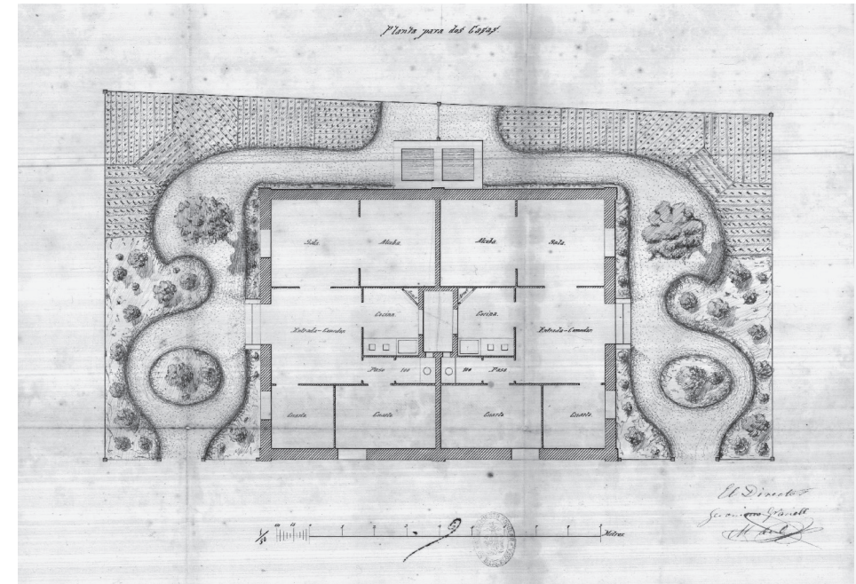
10. Planta de les dues cases per a obrers amb els jardins. Arxiu de la Societat Econòmica Barcelonesa d'Amics del País, 1874.
