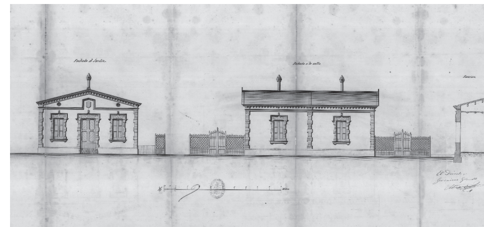
11. Façana des del carrer d'Urgell i alçat de les cases per a obrers. Arxiu de la Societat Econòmica Barcelonesa d'Amics del País, 1874.
